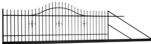
Brama przesuwna z zamkiem hakowym Szer. 4,00 m x Wys. 1,20 - 1,50 m L nr: 624332 Szer. 5,00 m x Wys. 1,20 - 1,50 m L nr: 634919 P nr: 624333 P nr: 634920 Z automatem L nr: 634949 Z automatem L nr: 634921 Z automatem P nr: 634950 Z automatem P nr: 634922
