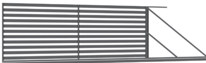
Brama przesuwna z automatem w słupku Szer. 4,00 m x Wys. 1,54 m L nr: 5903641455091 P nr: 5903641455107
